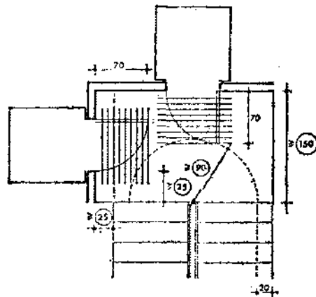
Meseta con desahogo de ascensor Plantas
