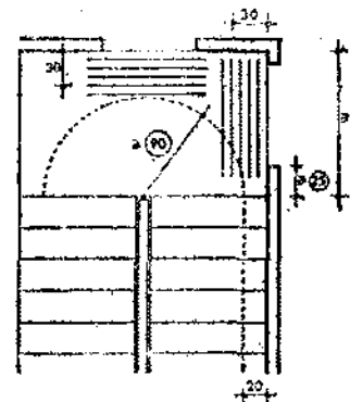
Meseta con planta a vigirala
