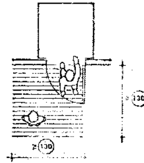
Espera ascensor en portal
