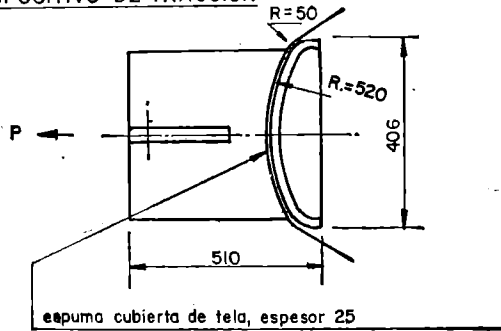
ANEXO 5 Fig. 1 DISPOSITIVO DE TRACCION
