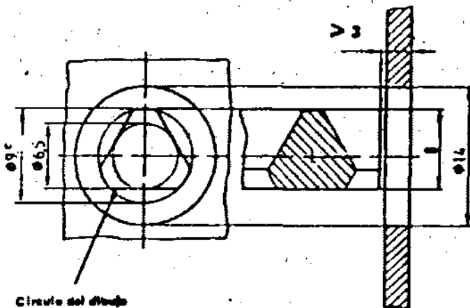
Fig. 4.- Triángulo de desenganamiento (cotas en milímetros)
