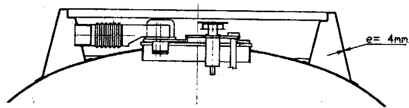
SECCION A-A
