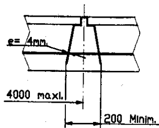
SECCION B-B
