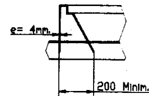
SECCION D-D
