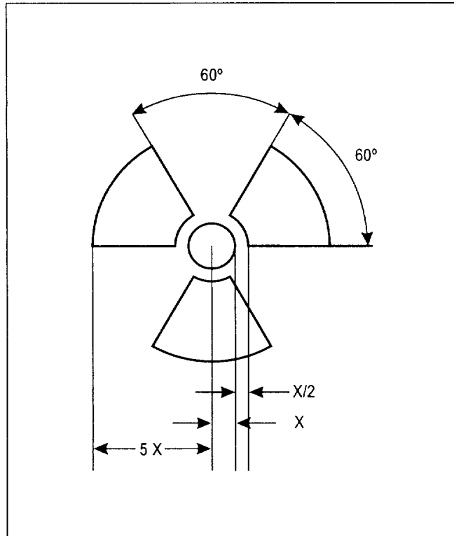
+ Figura 5.1 Símbolo del trébol esquematizado con las proporciones que corresponden a un círculo central de radio X. La dimensión mínima admisible debe ser de 4 mm.
