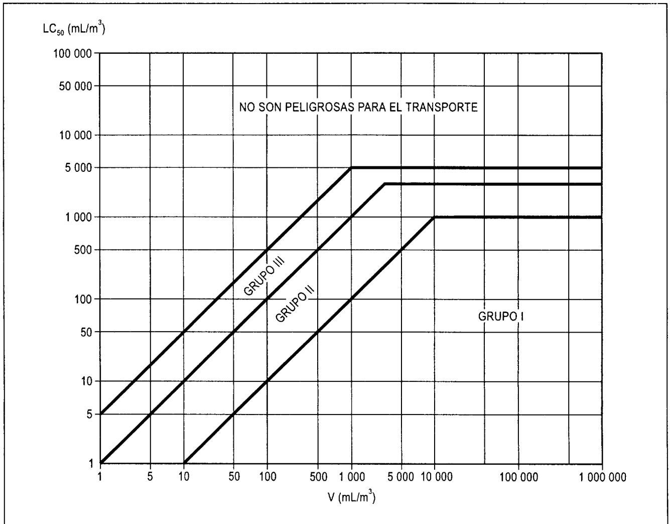
Figura 2-1. Criterios aplicables a la inhalación de vapores
