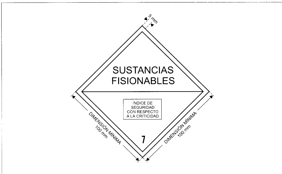
≠ Figura 5-19. Etiqueta para el índice de seguridad con respecto a la criticidad
