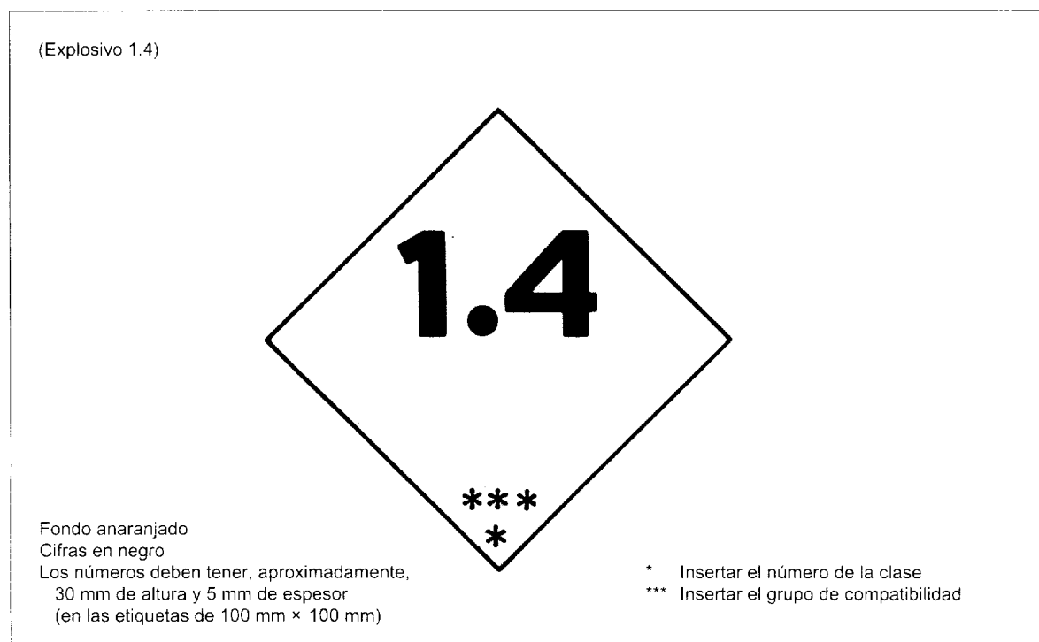
≠ Figura 5-3. Explosivo, Clase 1, División 1.4
