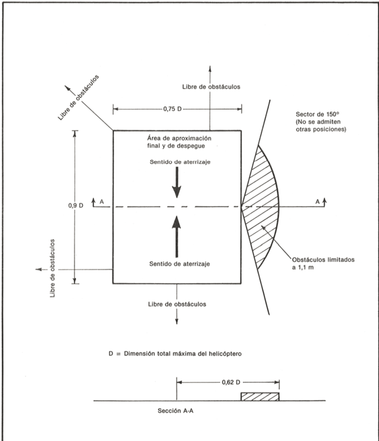
Figura 4-5. Sectores limitadores de obstáculos en la heliplatforma Helicópteros de rotor principal en tándem — Operaciones bidireccionales
