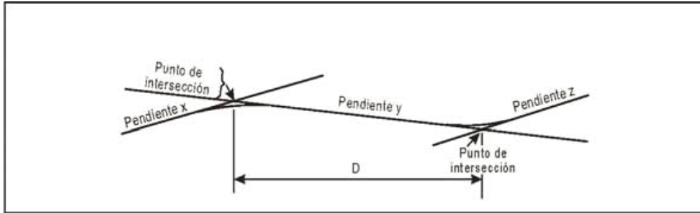
Figura A-2. Perfil del eje de la pista
