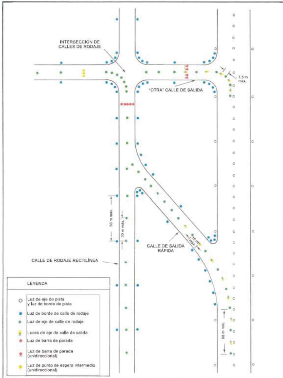
Figura 5-24. Iluminación de calles de rodaje
