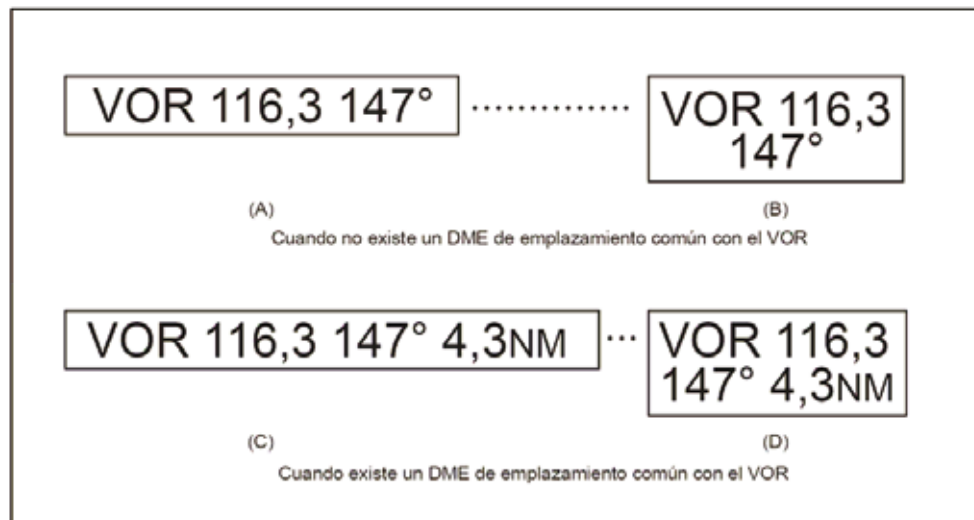
Figura 5-31. Letreros de punto de verificación del VOR en el aeródromo
