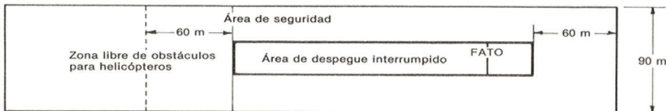
Figura 3-1. Área de seguridad de la FATO para aproximaciones por instrumentos
