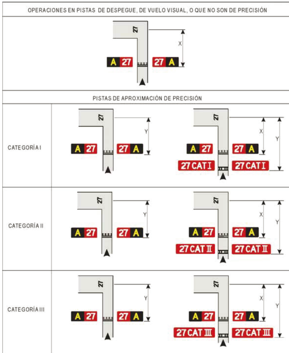
Figura 5-30. Ejemplos de la ubicación de los letreros en las intersecciones de calle de rodaje/pista
