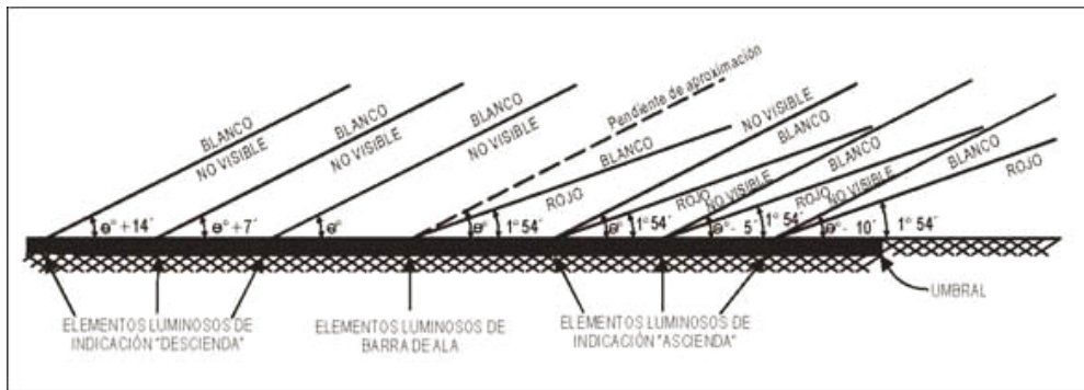
Figura 5-17. Haces luminosos y reglaje del ángulo de elevación del T-VASIS y del AT-VASIS
