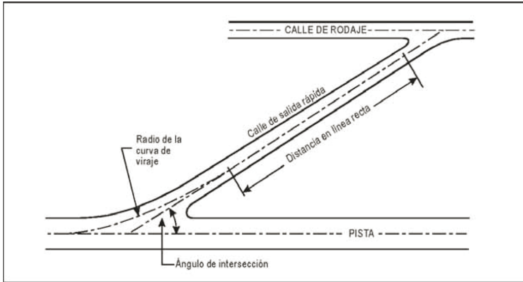
Figura 3-3. Calle de salida rápida
