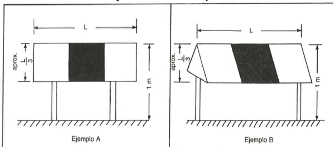
Figura 5-7. Baliza de ruta de desplazamiento aéreo
