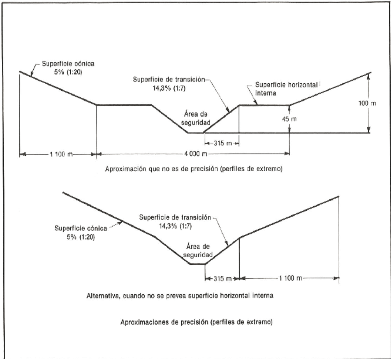
Figura 4-10. Superficies limitadoras de obstáculos de transición, horizontal interna y cónica
