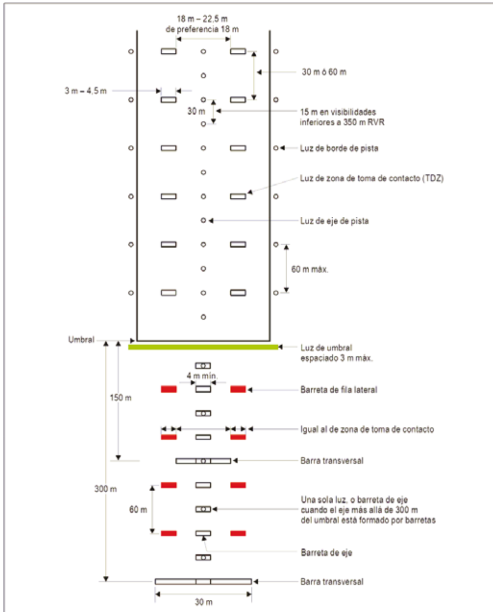
Figura 5-14. Iluminación de pista y de los 300 m internos de la aproximación, en las pistas para aproximaciones de precisión de Categorías II y III, cuando pueda demostrarse que se cumplen los niveles de funcionamiento de las luces especificados como objetivos de mantenimiento en el Capítulo 10
