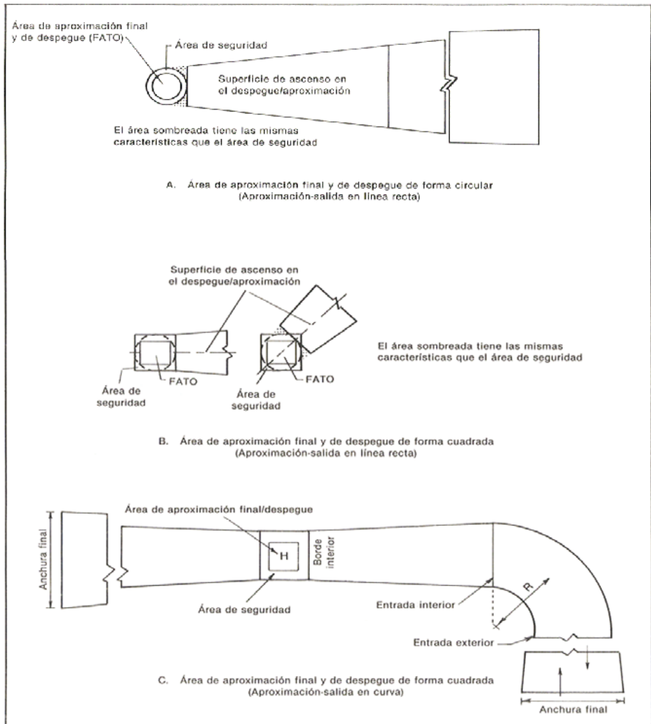
Figura 4-6. Superficie de ascenso en el despegue/aproximación (FATO para vuelo visual)
