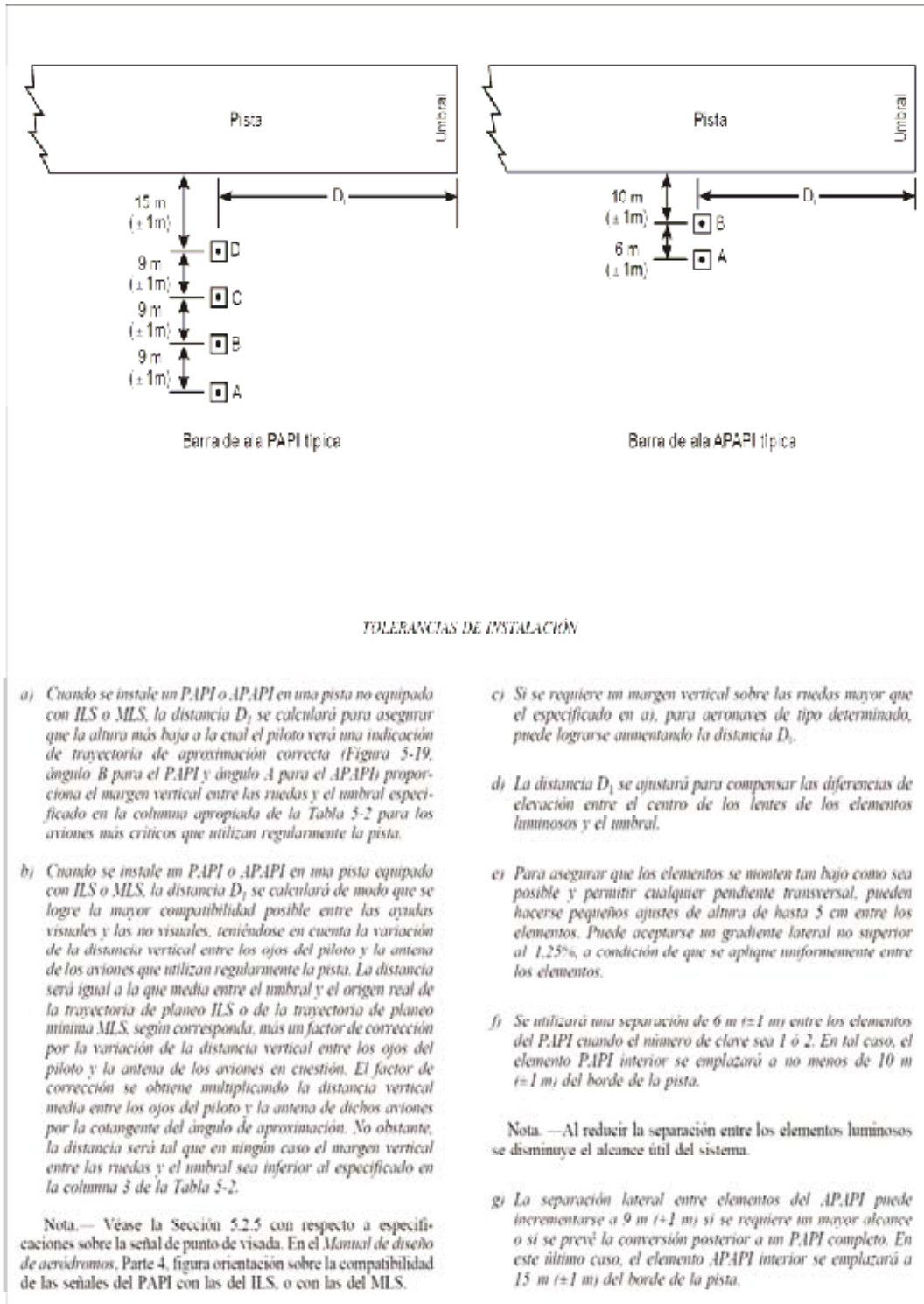
Figura 5-18. Emplazamientos del PAPI y del APAPI
