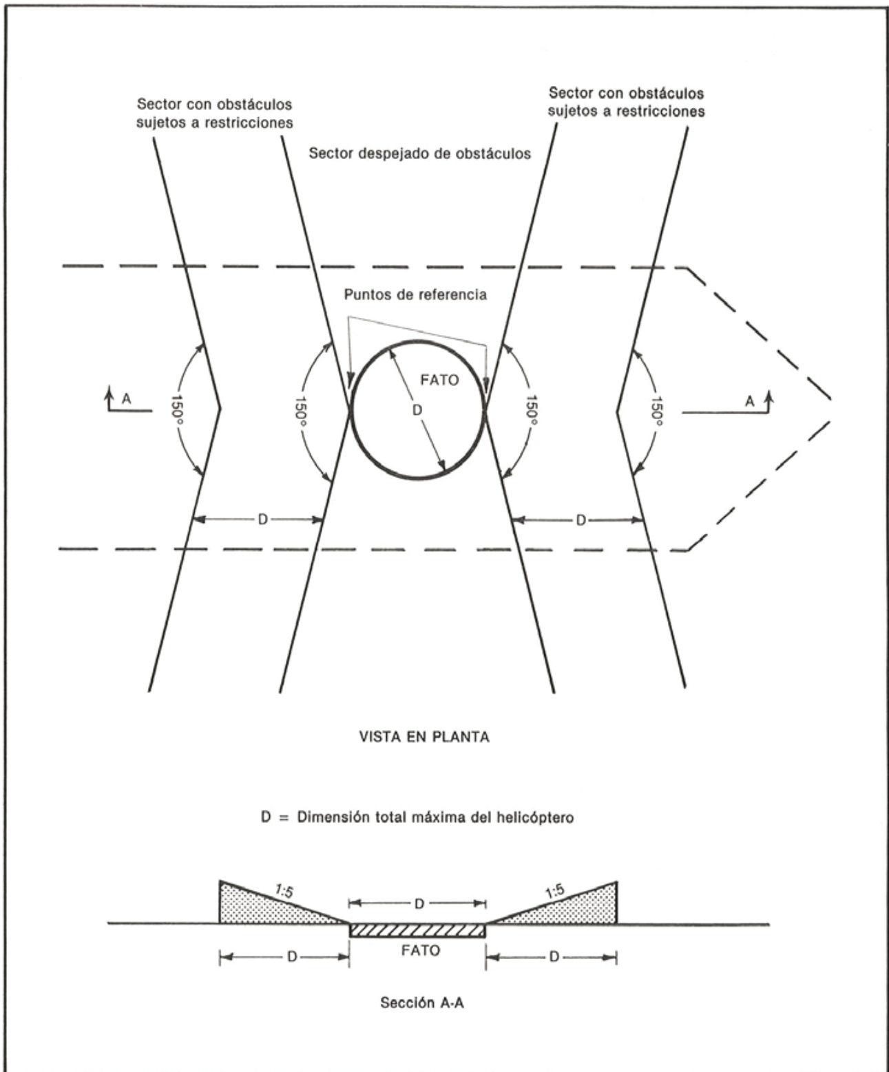
Figura 4-11. Superficies limitadoras de obstáculos en los helipuertos no construidos para fines especiales en el centro del buque
