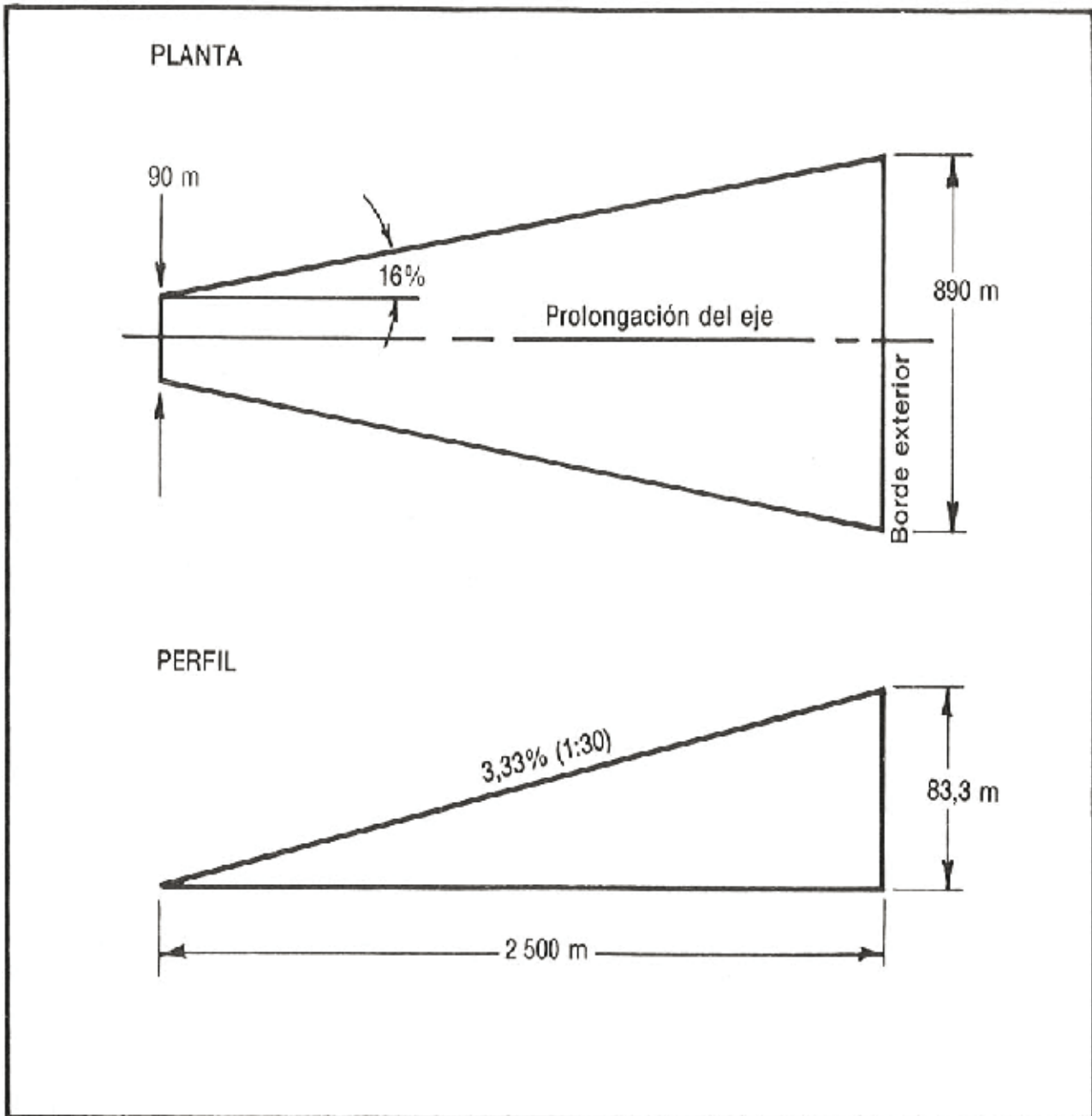
Figura 4-9. Superficie de aproximación de la FATO para aproximaciones que no sean de precisión
