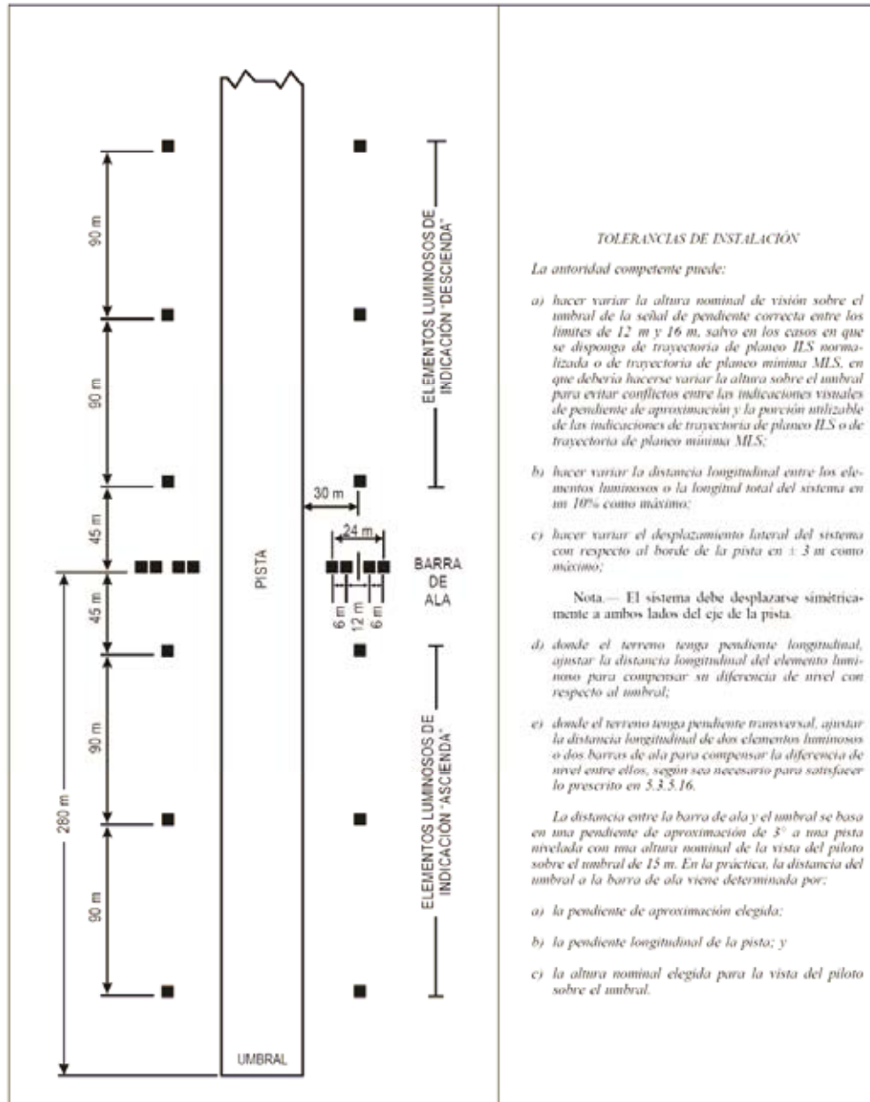
Figura 3-16. Emplazamiento de los elementos luminosos del T-VASIS
