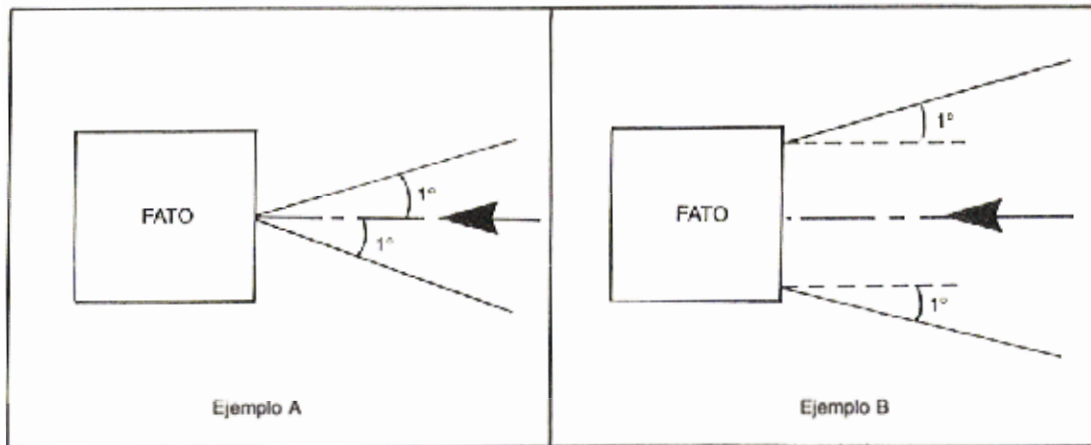
Figura 5-11. Divergencia del sector "derrota correcta"
