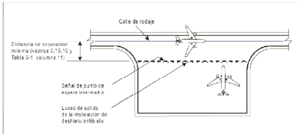
Figura 5-26. Típica instalación de deshielo/antihielo distante
