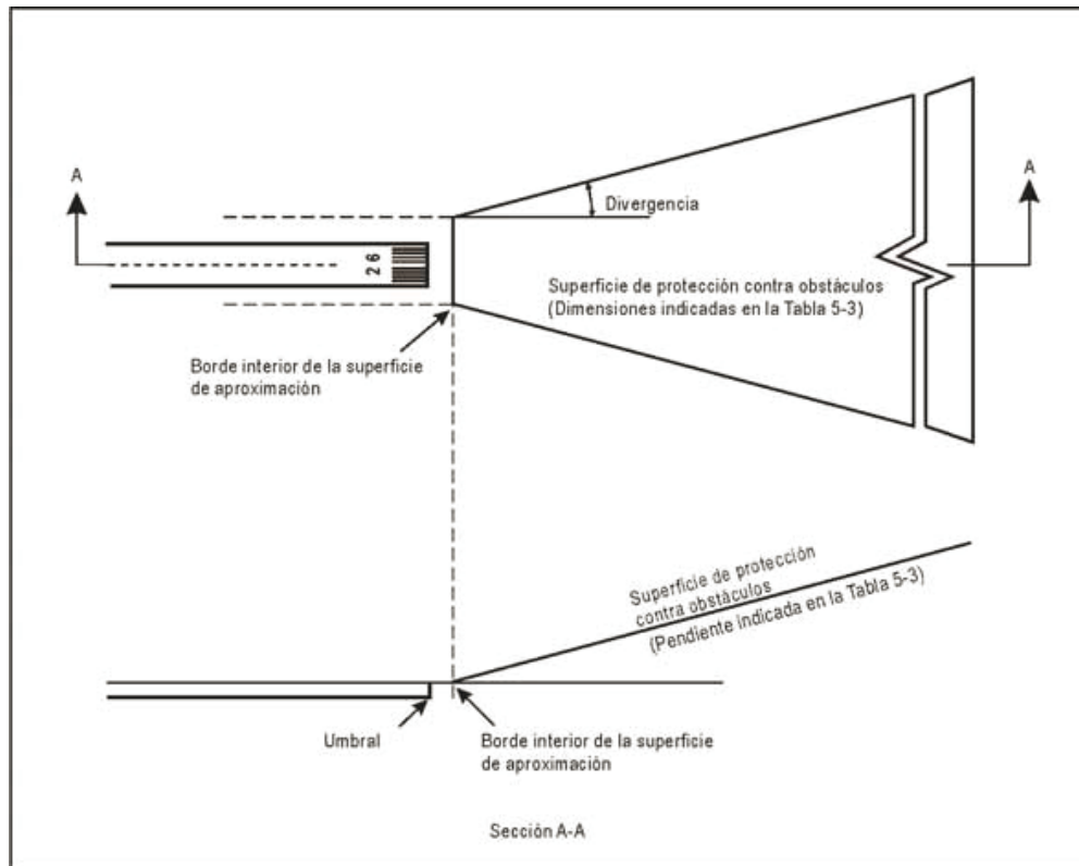
Figura 5-20. Superficie de protección contra obstáculos para los sistemas visuales indicadores de pendiente de aproximación
