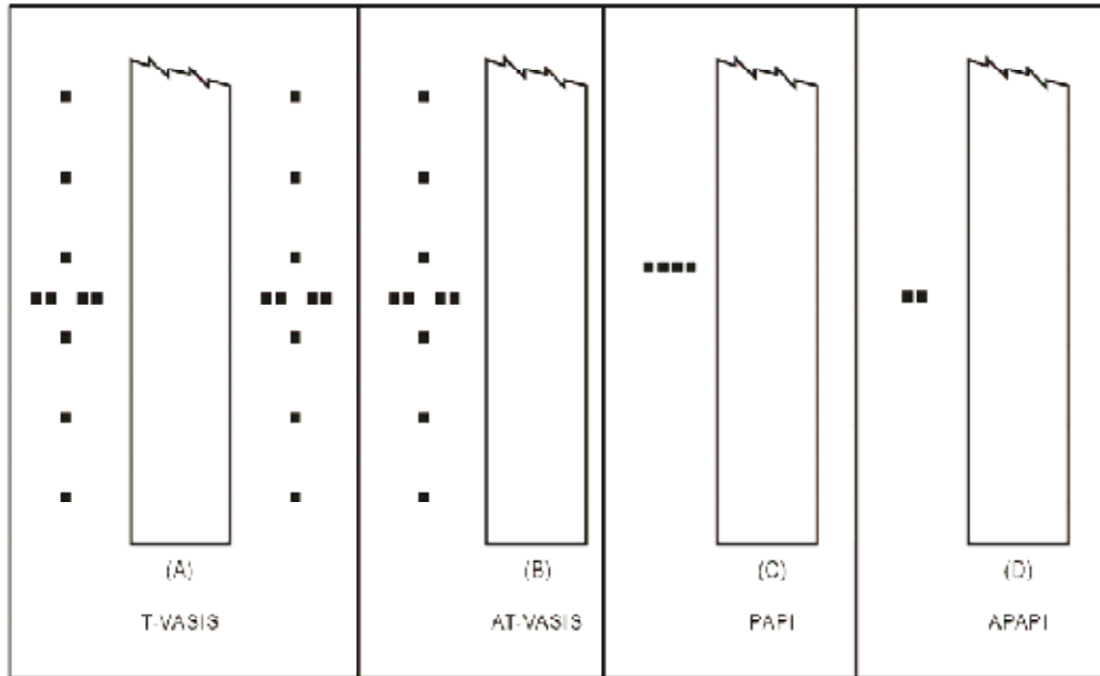
Figura 5-15. Indicadores visuales de pendiente de aproximación
