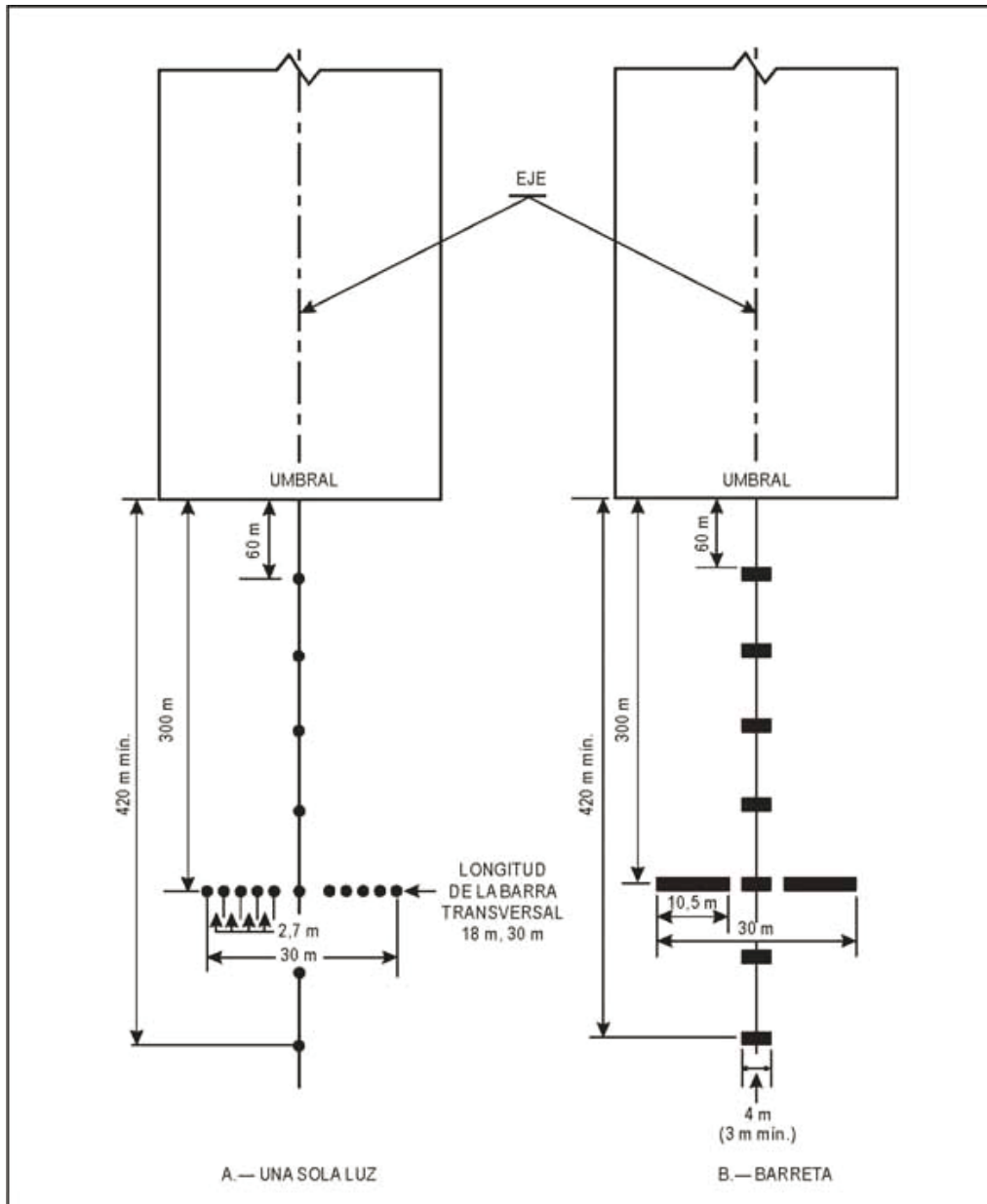
Figura A-5. Sistemas sencillos de iluminación de aproximación
