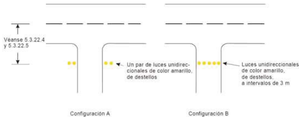
Figura 5-27. Luces de protección de pista
