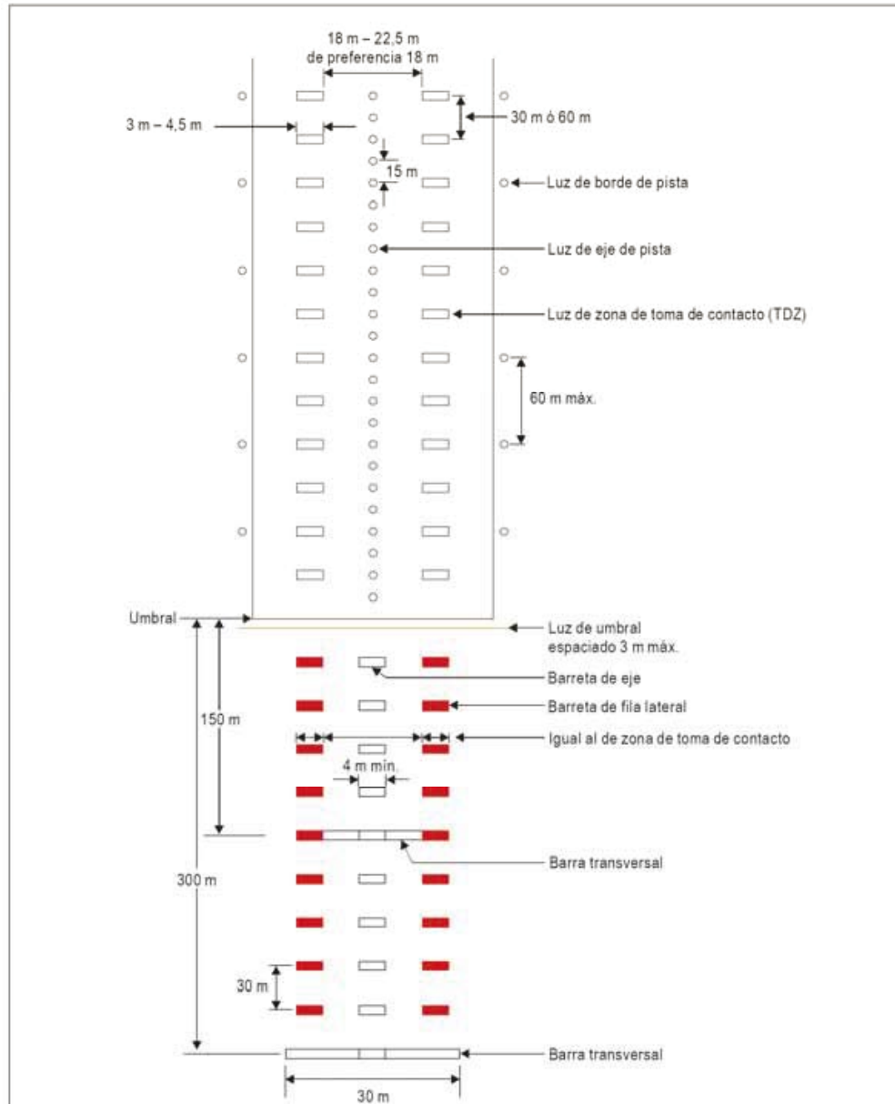
Figura 5-13. Iluminación de pista y de los 300 m internos de la aproximación, en las pistas para aproximaciones de precisión de Categorías II y III
