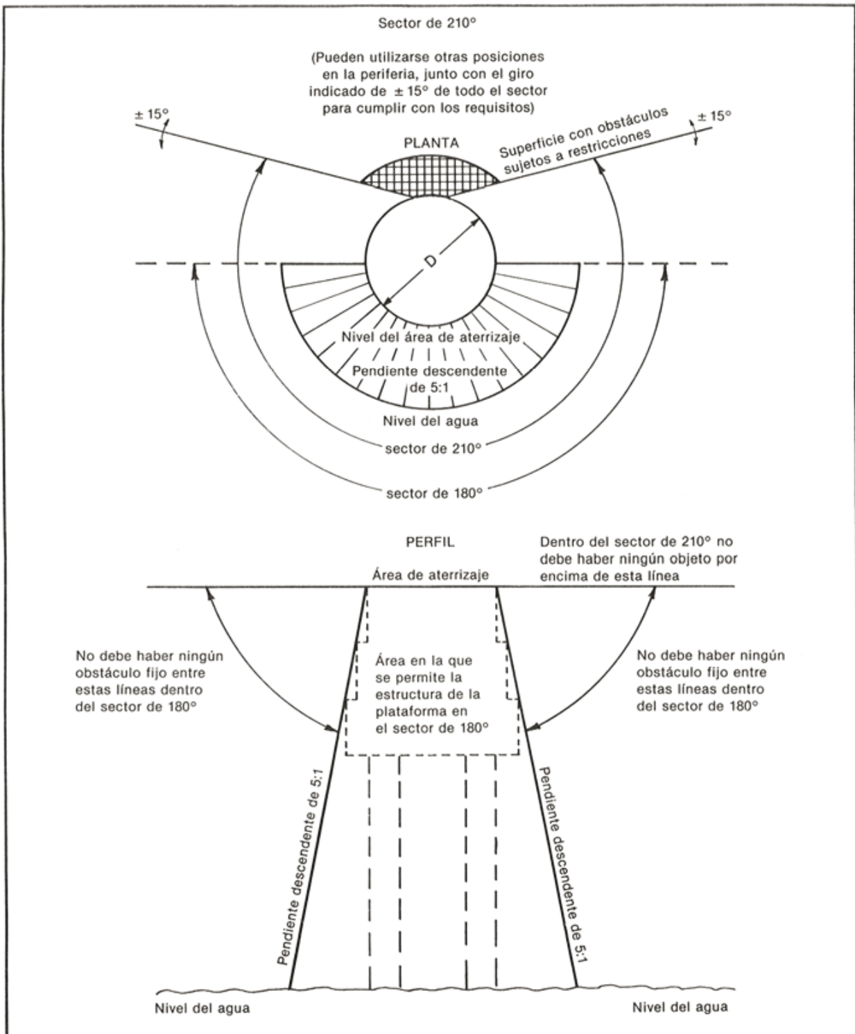
Figura 4-2. Sector libre de obstáculos de la heliplataforma
