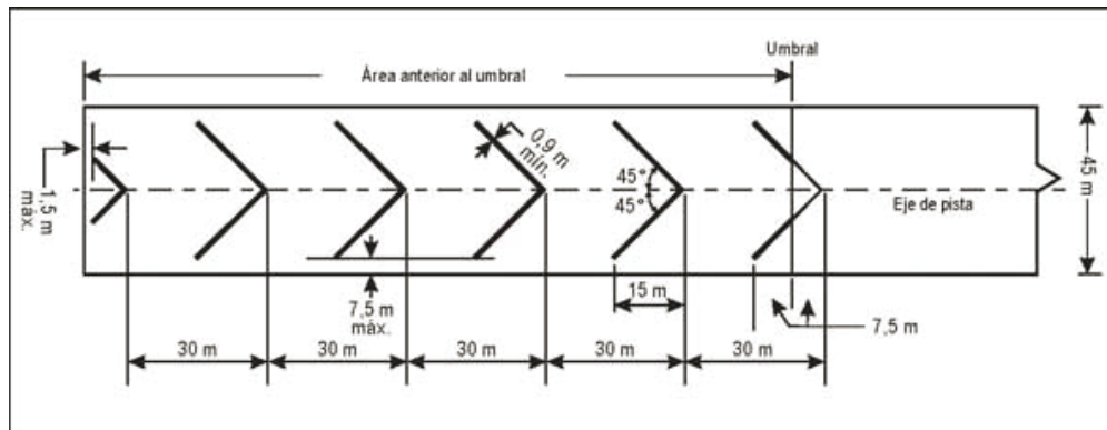
Figura 7-2. Señal anterior al umbral
