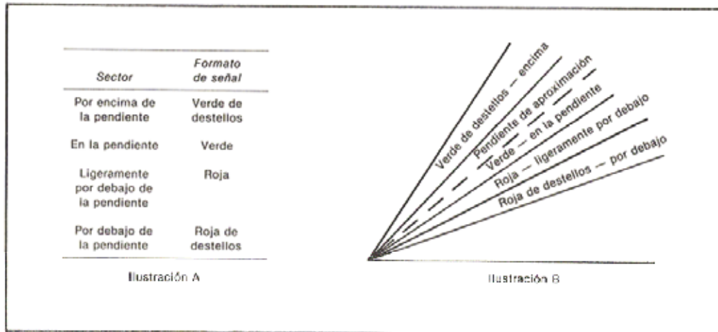
Figura 5-12. Formato de la señal HAPI
