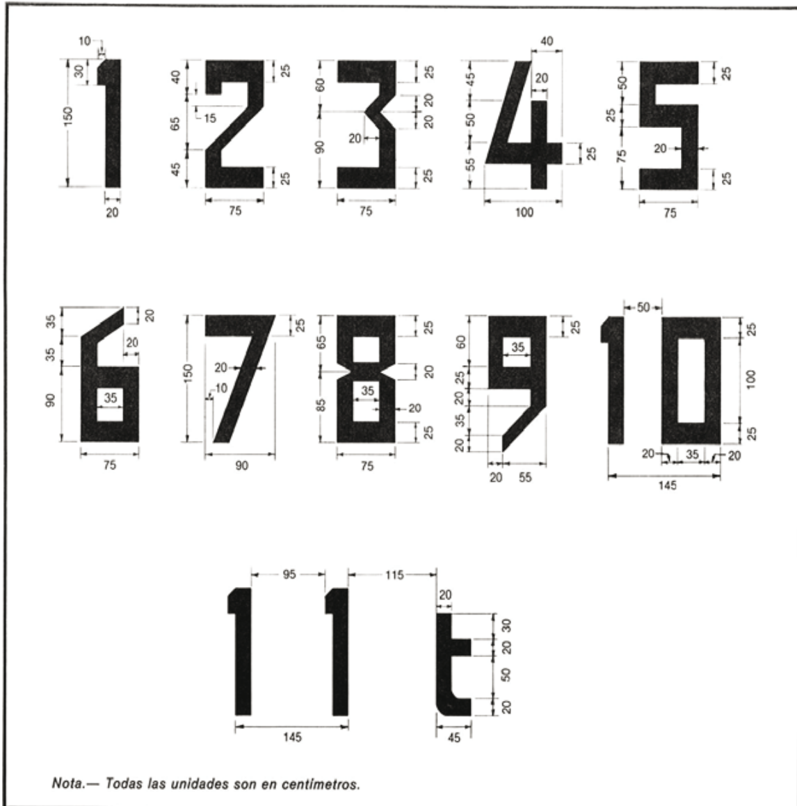
Figura 5-2. Forma y proporciones de los números y de la letra de la señal de masa máxima permisible
