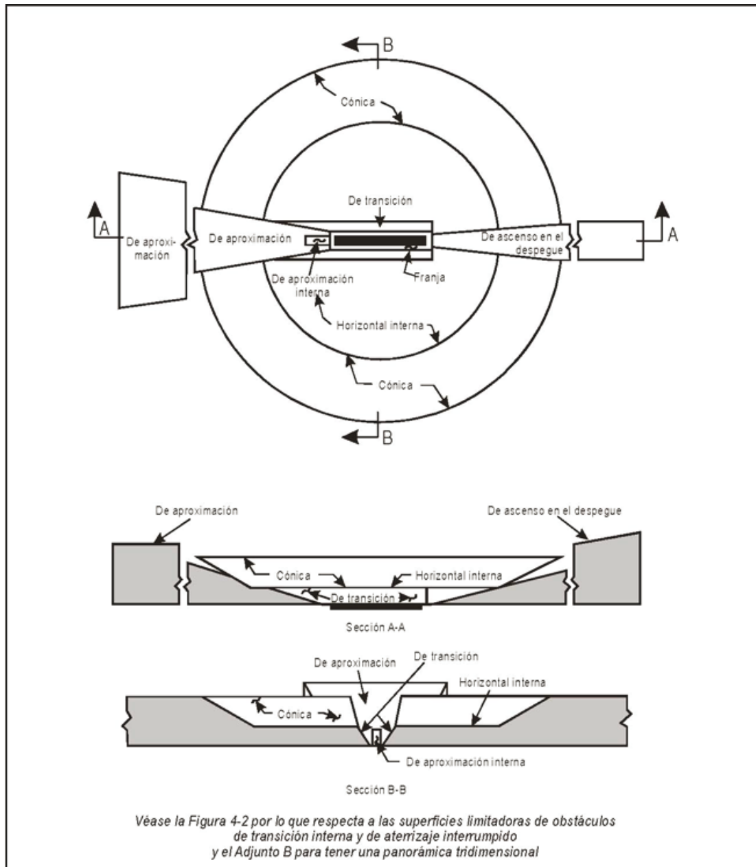
Figura 4-1. Superficies limitadoras de obstáculos
