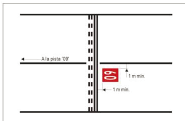
Figura 5-9. Señal con instrucciones obligatorias
