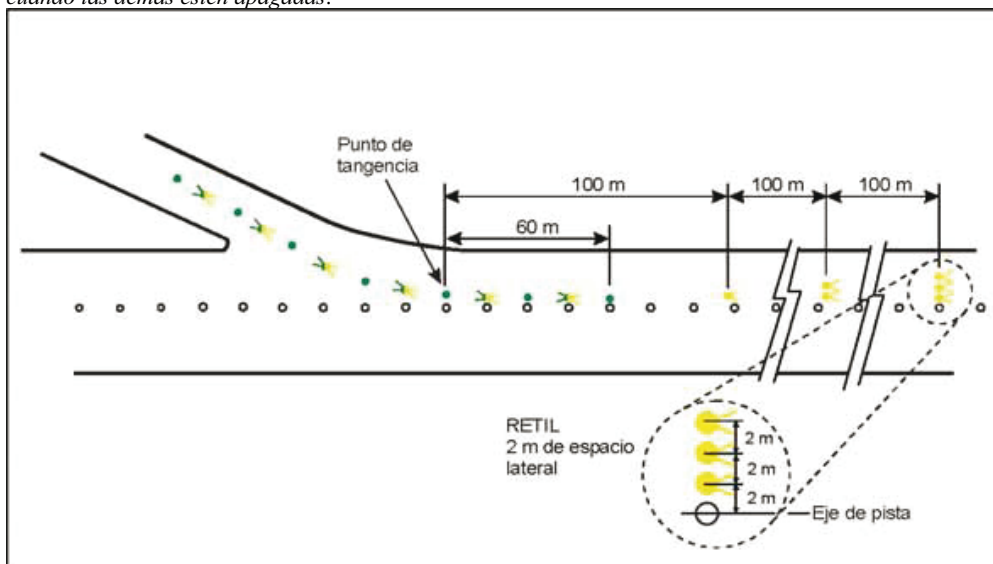
Figura 5-23. Luces indicadoras de calle de salida rápida
