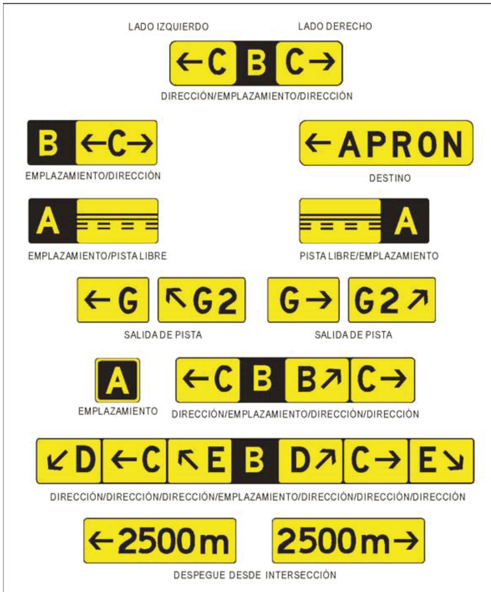
Figura 5-29. Letreros de información
