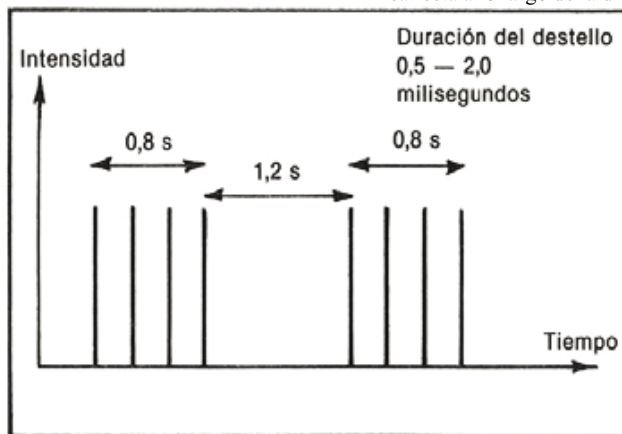
Figura 5-8. Características de los destellos de un faro de helipuerto
