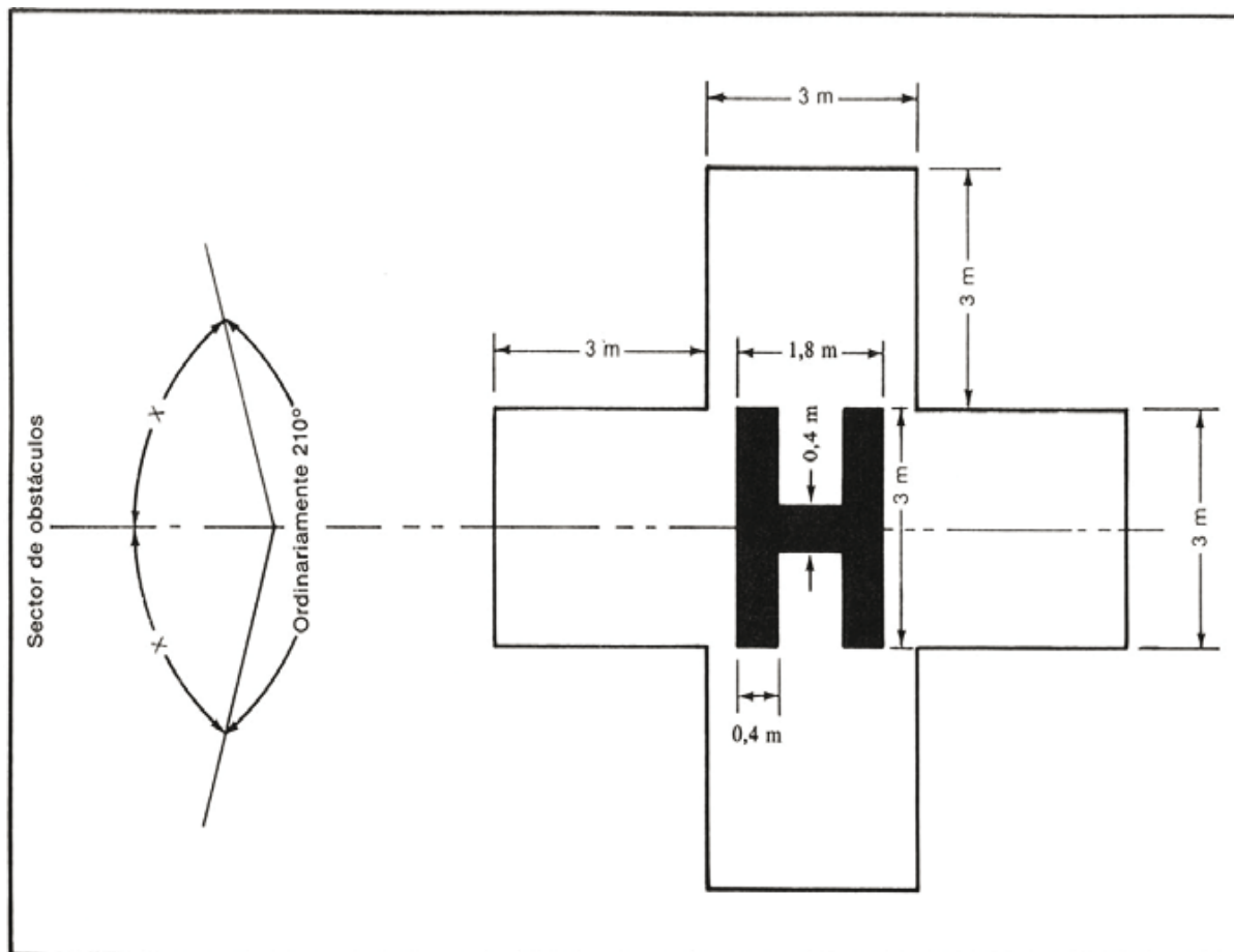
Figura 5-1. Señal de identificación de helipuerto (indicada con una cruz de hospital y orientada con el sector despejado de obstáculos)
