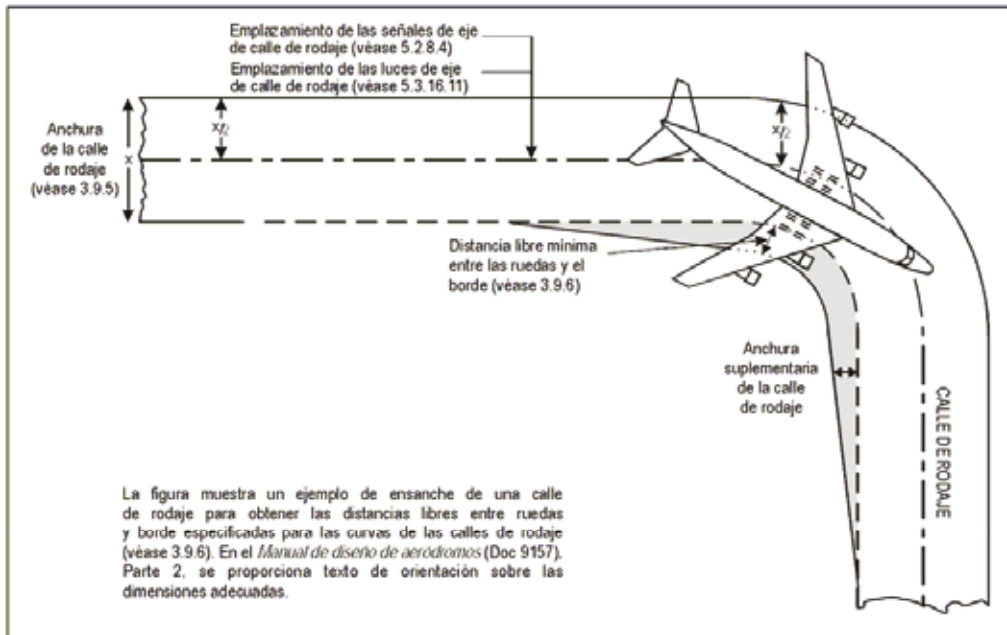
Figura 3-2. Curva de calle de rodaje
