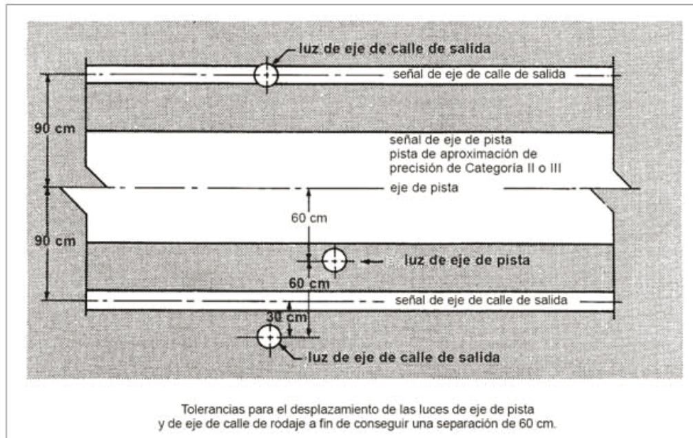
Figura 5-25. Desplazamiento de las luces de eje de pista y de eje de calle de rodaje
