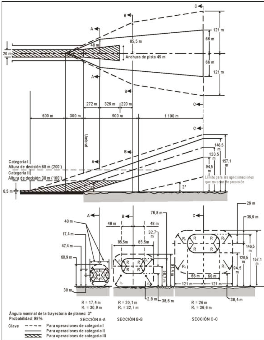
Figura A-4. Envolventes de trayectorias de vuelo que han de utilizarse en el proyecto de iluminación para las operaciones de las Categorías I, II y III
