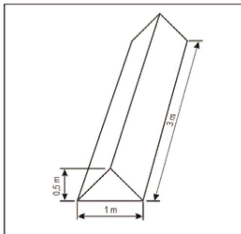
Figura 5-32. Balizas delimitadoras
