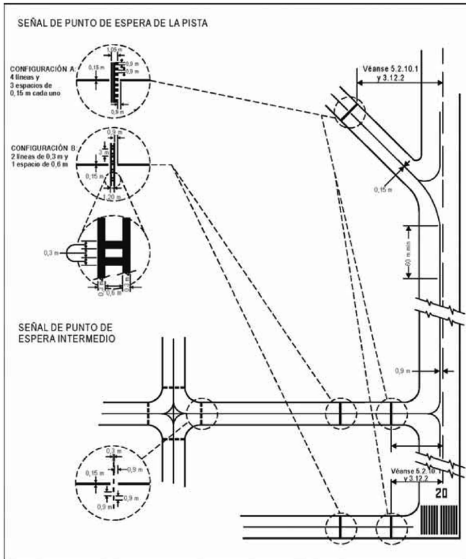
Figura 5-6. Señales de calle de rodaje
