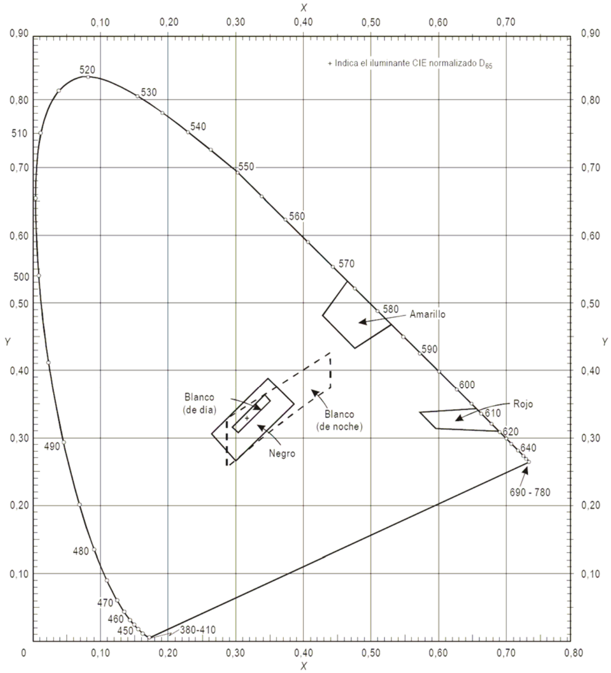
Figura A1-4. Colores de los letreros y paneles transluminados (iluminación interna)
