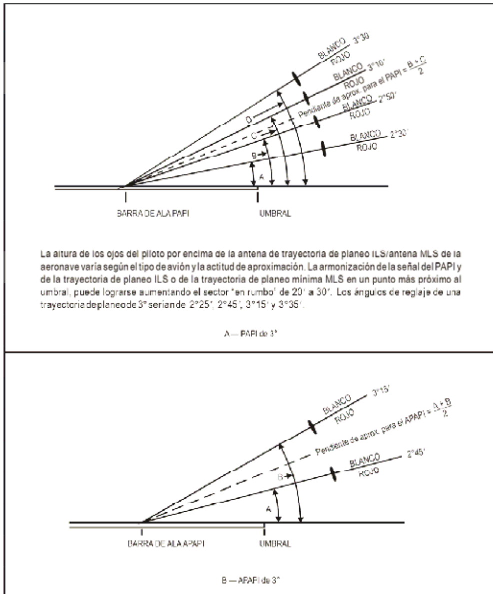
Figura 5-19. Haces luminosos y reglaje del ángulo de elevación del PAPI y del APAPI
