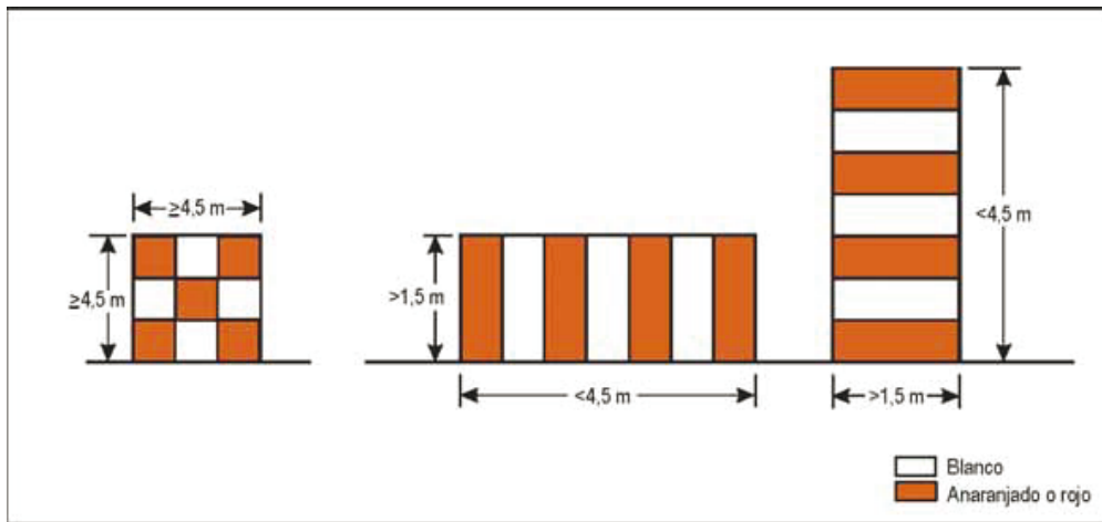
Figura 6-1. Configuraciones básicas del señalamiento de obstáculos
