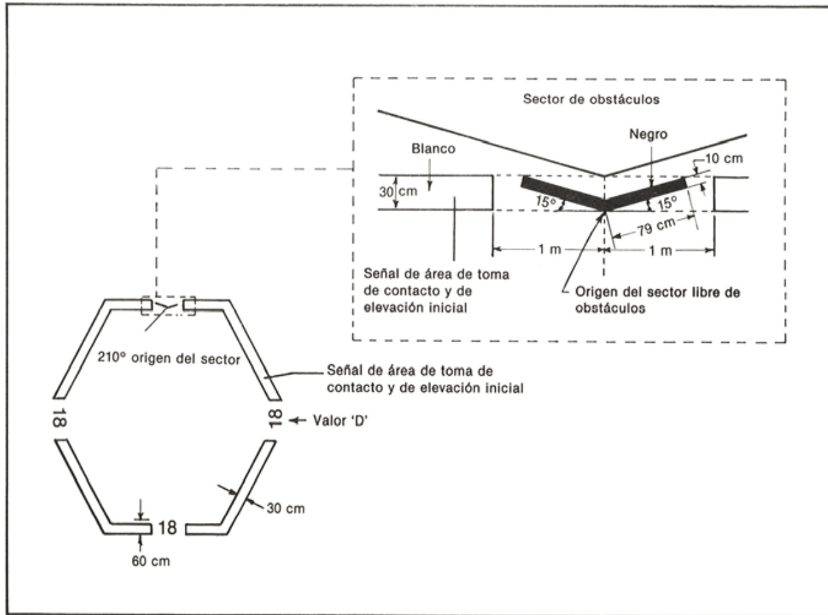
Figura 5-5. Señal de sector despejado de obstáculos de heliplataforma
