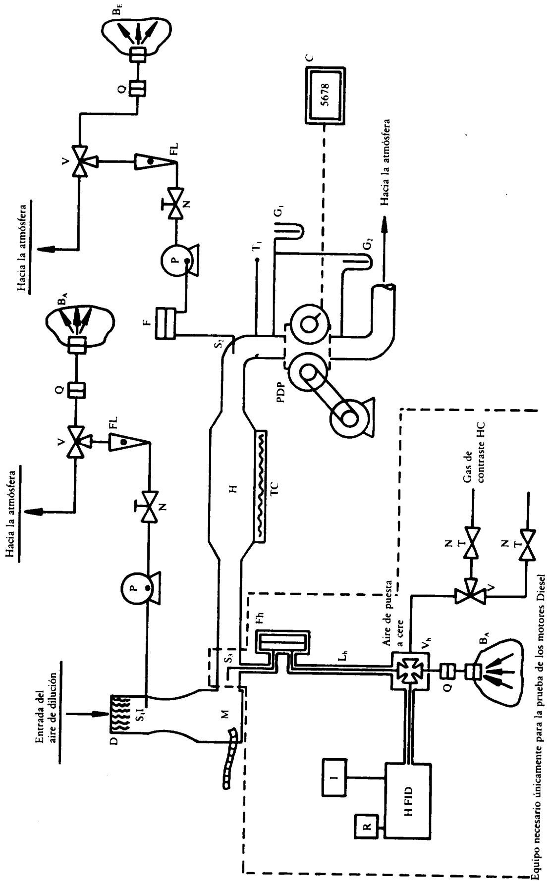
Figura 1 Esquema de un sistema de toma de muestras de volumen constante con bomba volumétrica (sistema PDP-CVS)
