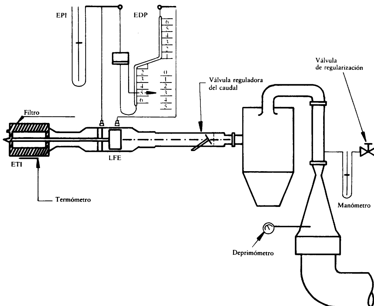
Configuración de calibrado para el sistema CFV-CVS
