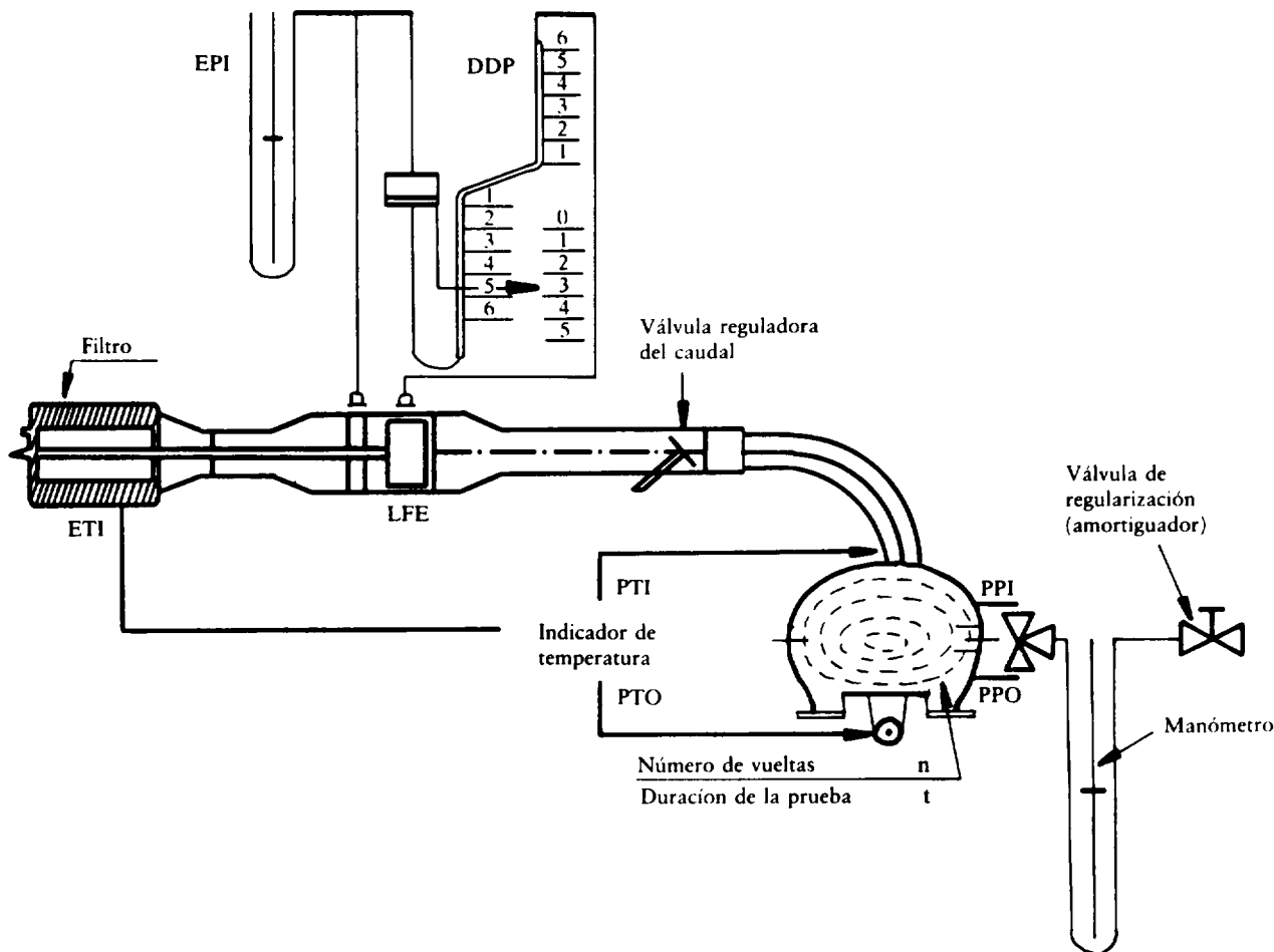
Configuración de calibrado para el sistema PDP-CVS
